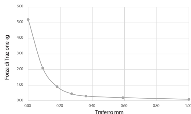
Elettromagnete di Tenuta: 20mm
