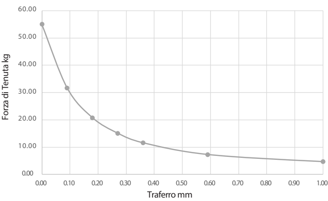
Magnete di Tenuta Elettropermanente: 50mm 24VDC
