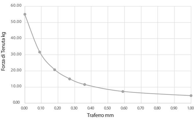
Magnete di Tenuta Elettropermanente: 50mm 240VAC
